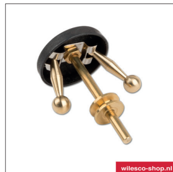
01619 Centrifugaalregelaar
