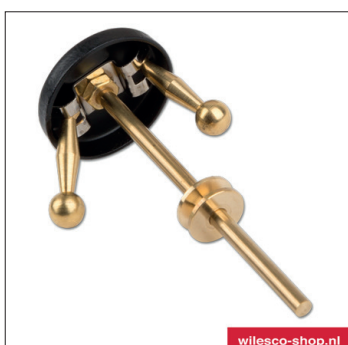
01620 Centrifugaalregelaar
